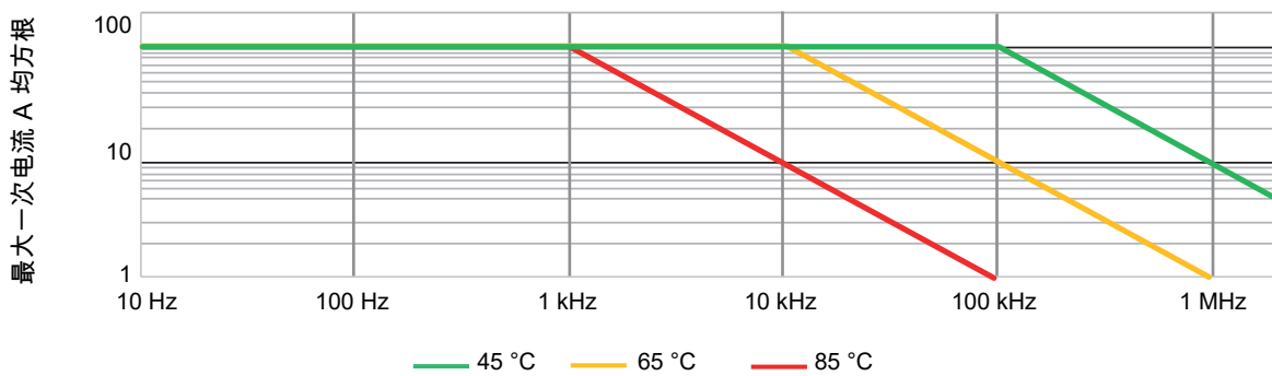
图 2: 频率和环境温度降额
