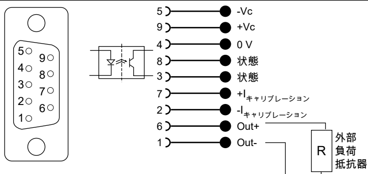
図 1.4: 標準 D-SUB 9 電流出力
