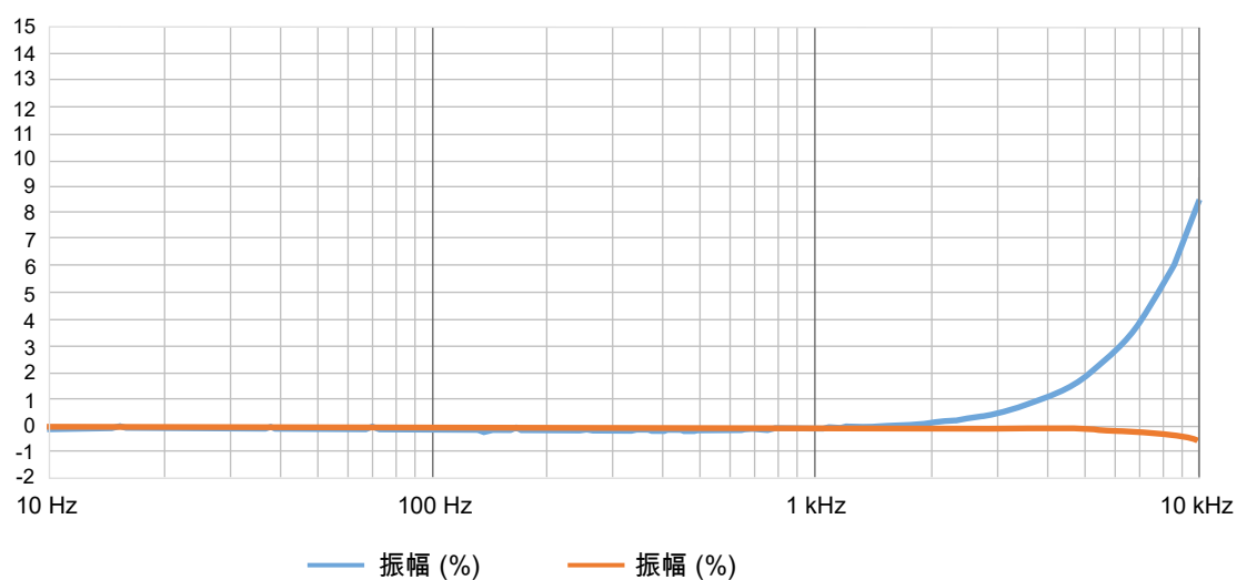
図 1.3: 周波数特性
