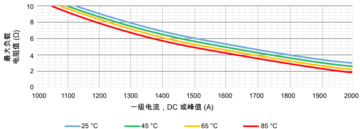
図 1.1: 負荷抵抗 RM および周囲温度ディレーティング
