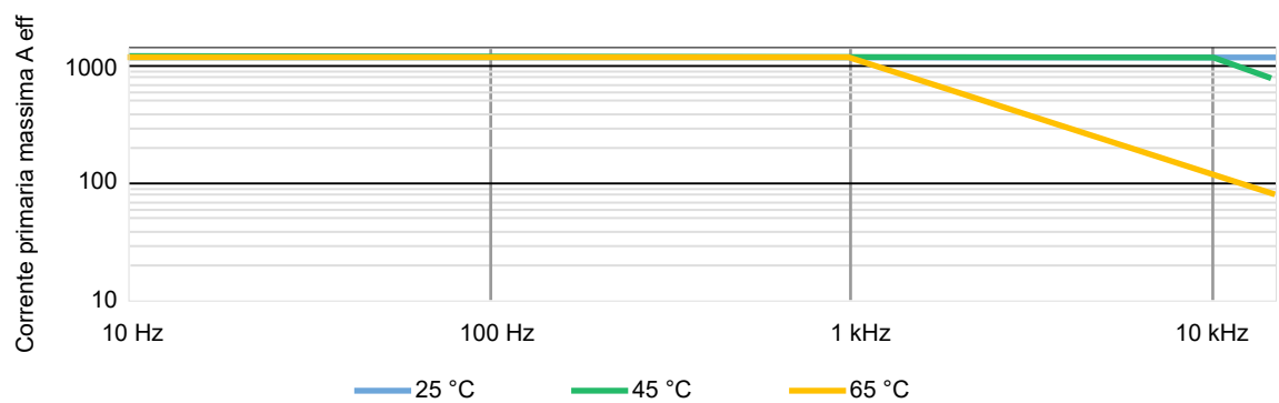
Figura 1.2: Derating di frequenza e temperatura ambientale
