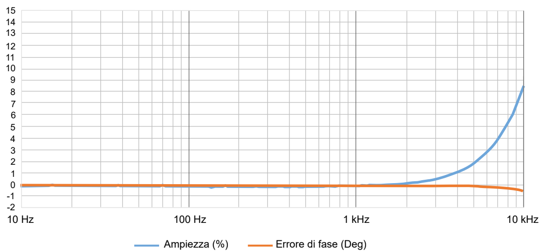
Figura 1.3: Dati caratteristici di frequenza
