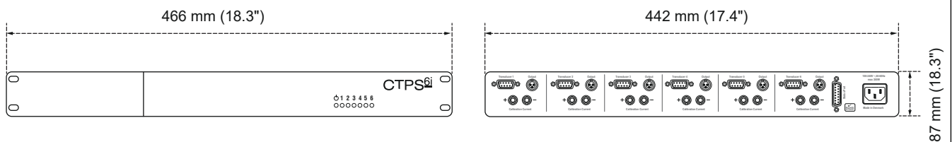
Figura 1.7: Dimensioni
