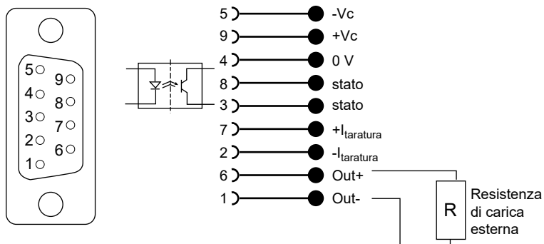
Figura 1.4: Uscita di corrente standard D-SUB 9
