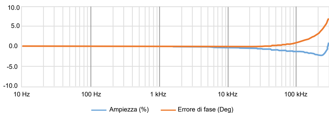
Figura 1.3: Dati caratteristici di frequenza
