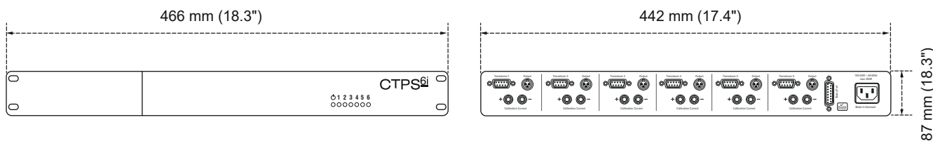
Figura 1.7: Dimensioni
