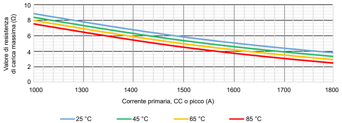
Figura 1.1: Resistenza di carica RM e derating temperatura ambientale
