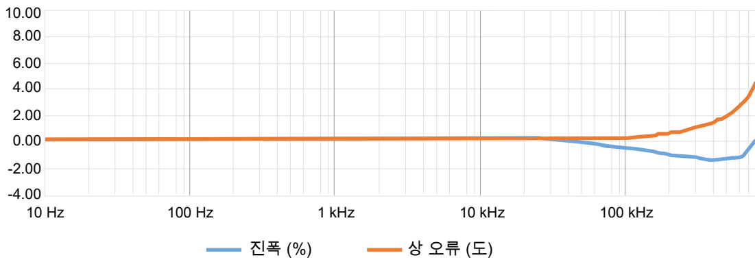
그림 1.3: 주파수 특성
