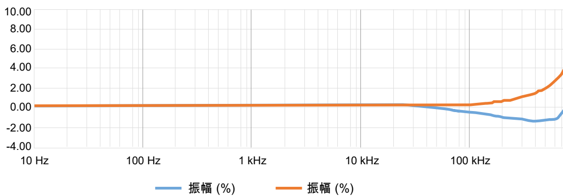
図 1.3: 周波数特性
