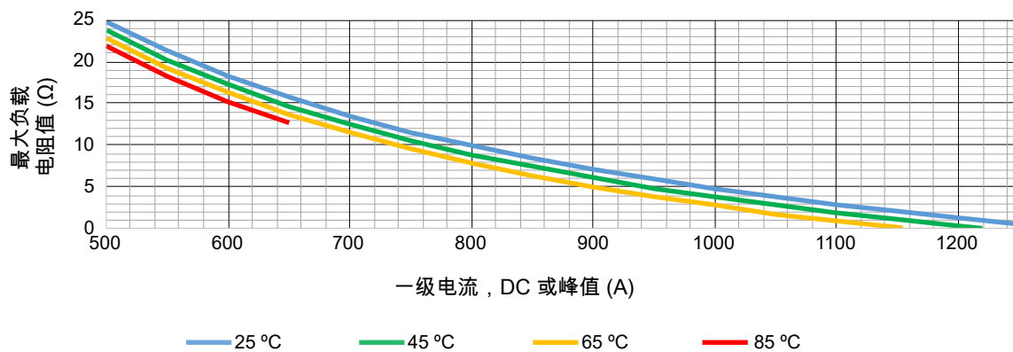
図 1.1: 負荷抵抗 RM および周囲温度ディレーティング
