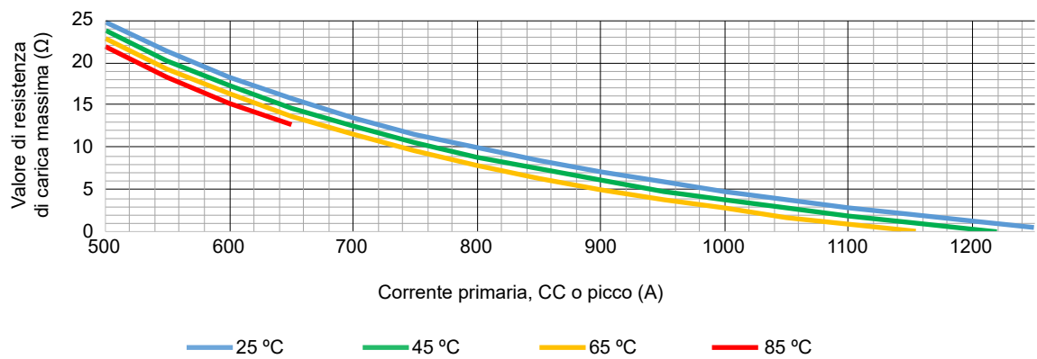
Figura 1.1: Resistenza di carica RM e derating temperatura ambientale
