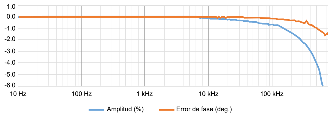
Figura 1.3: Características de frecuencia
