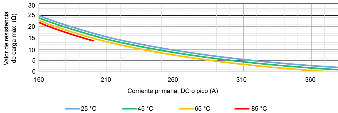
Figura 1.1: Resistencia de carga RM y reducción (derating) de la temperatura ambiente
