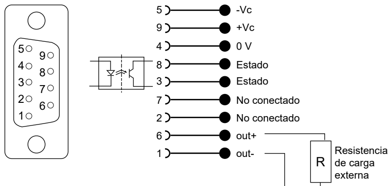
Figura 1.4: Salida de corriente del D-SUB 9 estándar
