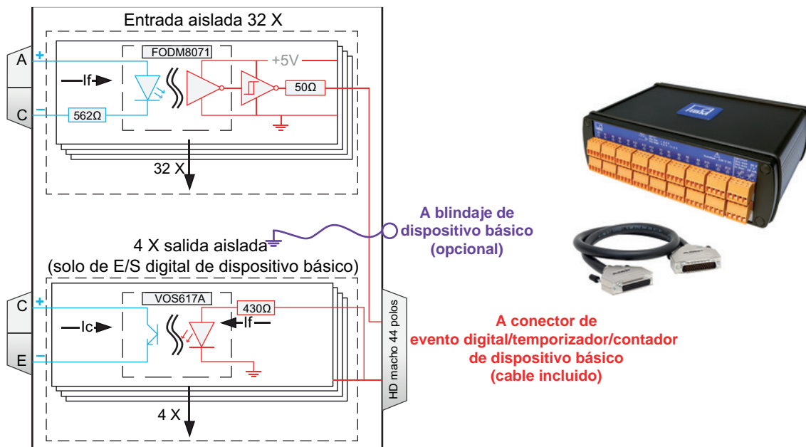
Figura 26: Diagrama de bloques y foto
