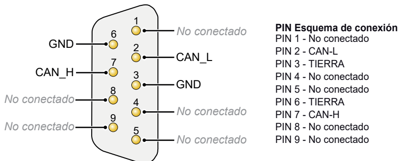
Figura 32: Esquema de conexión D-Sub
