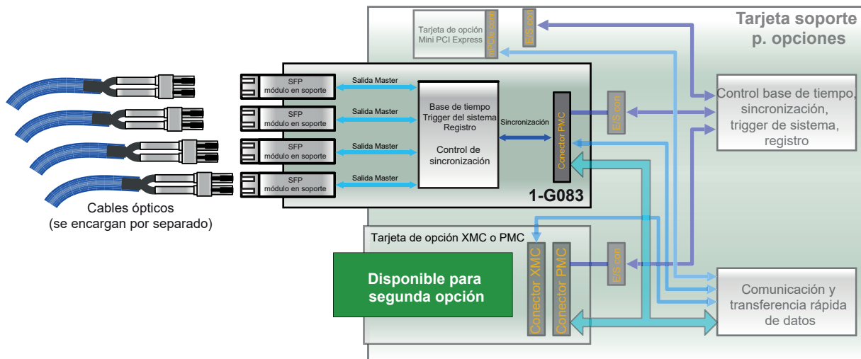
Figura 21: Diagrama de bloques de la tarjeta de salida master (opción G081 requerida)
