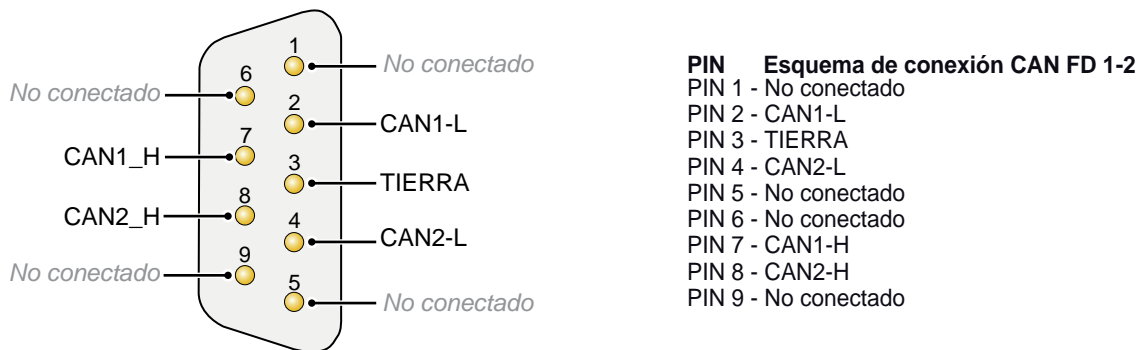
Figura 30: Esquema de conexión opción CAN FD
