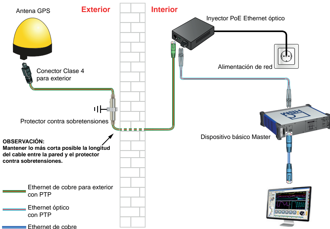
Figura 28: Ejemplo de configuración de la sincronización de hora GPS
