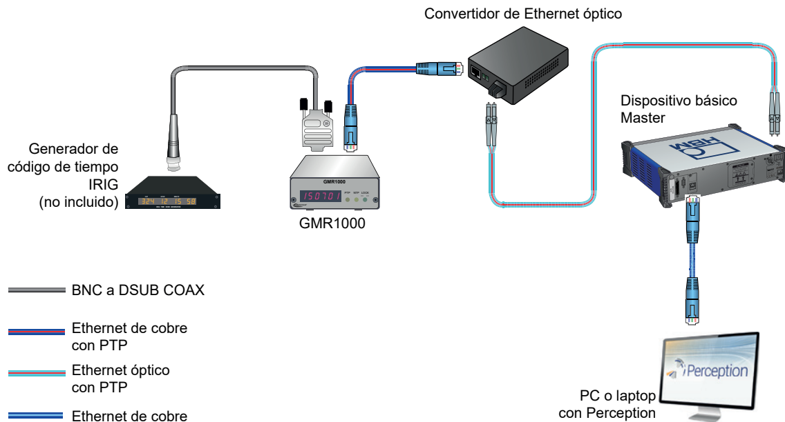
Figura 27: Ejemplo de configuración de la sincronización horaria IRIG
