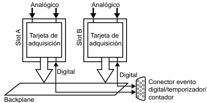
Figura 15: Diagrama de bloques de Evento digital/Temporizador/Contador
