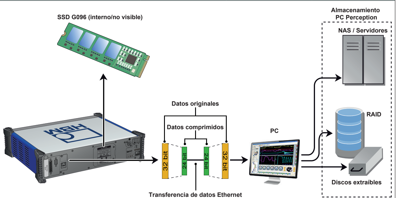
Figura 11: Vista de conjunto del streaming continuo
