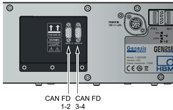
Figura 29: GEN2tB con CAN FD instalado en parte superior (detalle)
