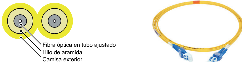
Figura 23: Diagrama de bloques y foto
