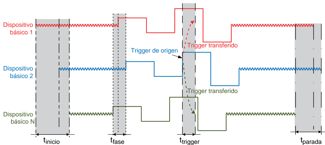
Figura 13: Vista de conjunto de las especificaciones de sincronización
