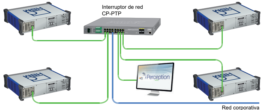
Figura 6: Dispositivos básicos múltiples (distribuidos)
