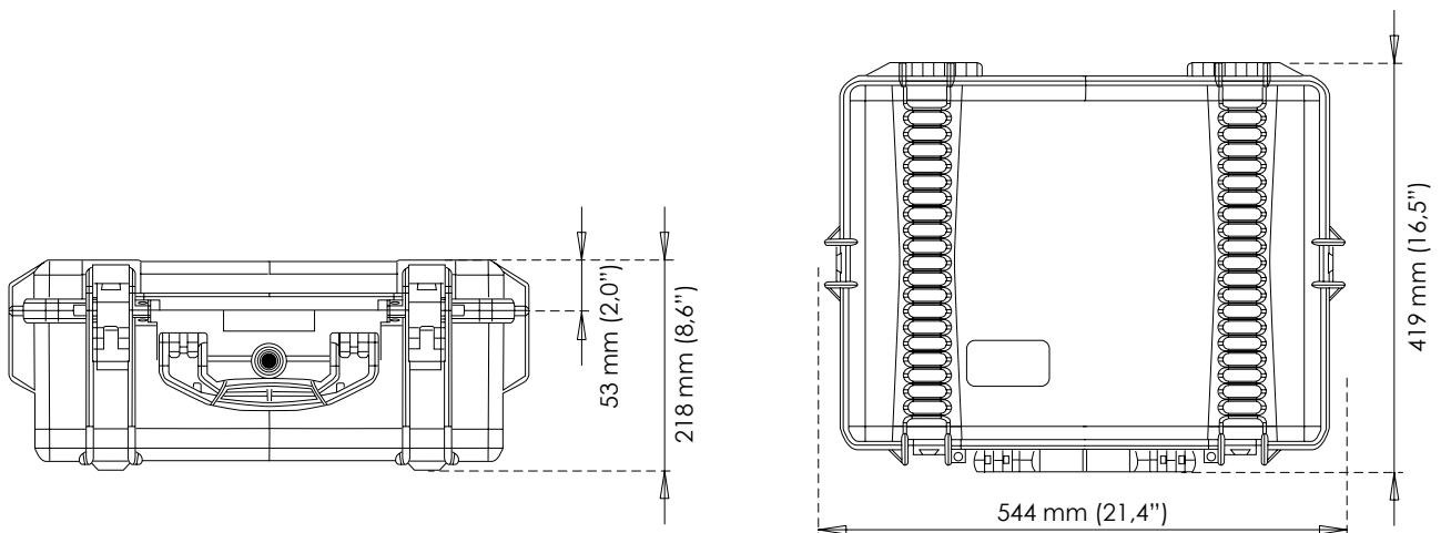
Figura 34: Maleta de transporte rígida reutilizable
