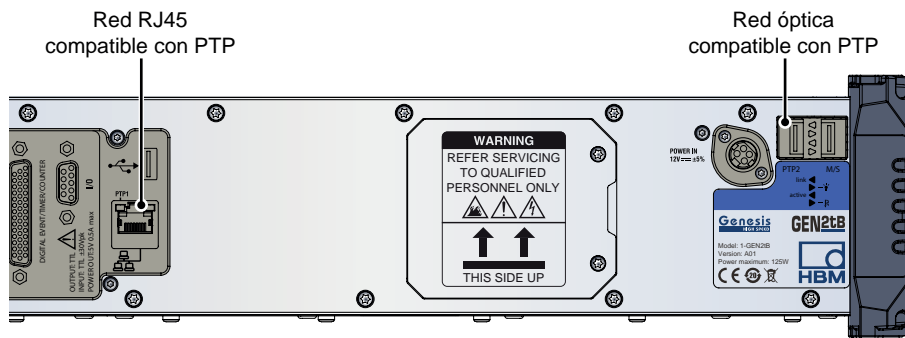
Figura 10: Interfaz de red eléctrica y de fibra óptica de 1 Gbit
