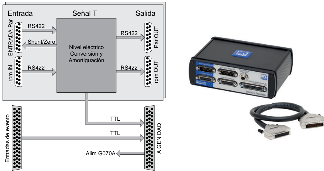
Figura 25: Diagrama de bloques y foto
