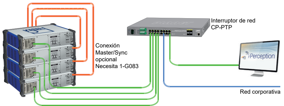
Figura 5: Dispositivos básicos múltiples
