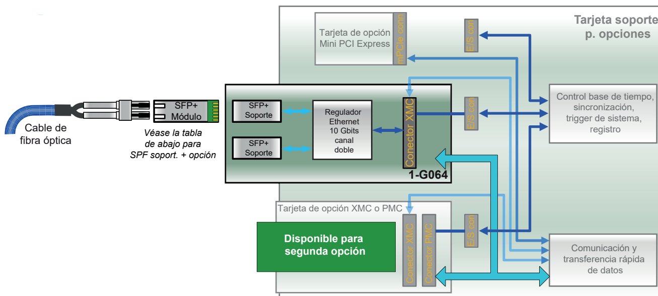
Figura 20: Diagrama de bloques de la tarjeta Ethernet de 10Gbit, fibra óptica (se requiere G081)
