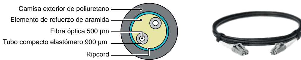
Figura 24: Diagrama de bloques y foto
