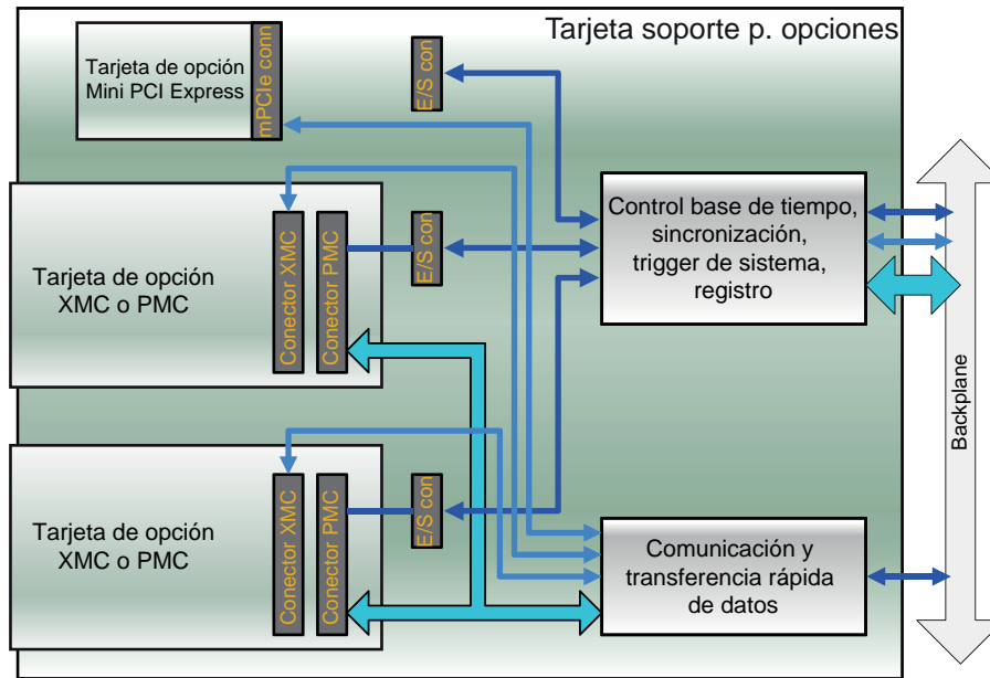
Figura 19: Diagrama de bloques de tarjeta soporte para opciones
