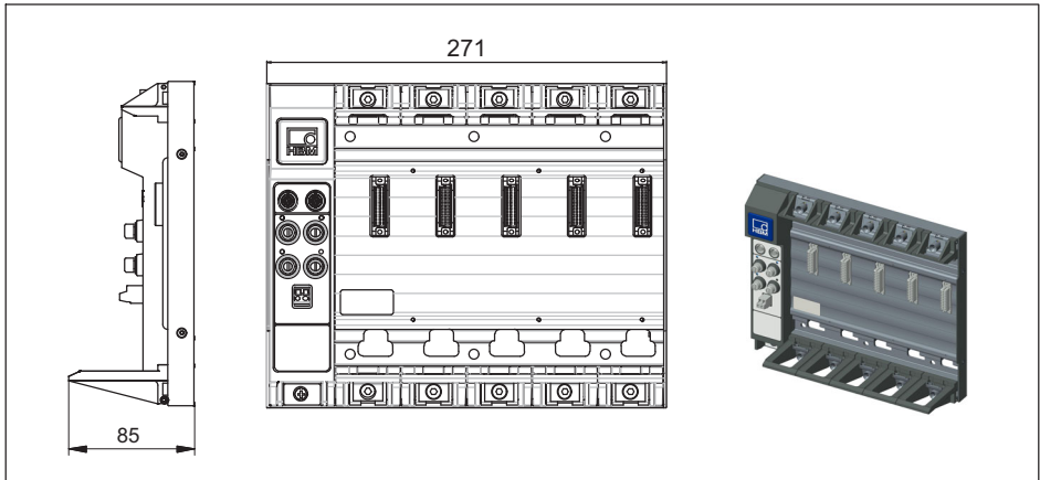
Fig. 6.15 BPX003 backplane
