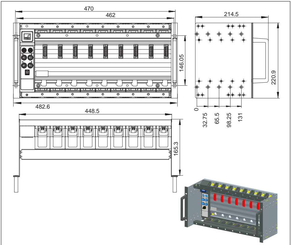
Fig. 6.14 Rackmontage BPX002
